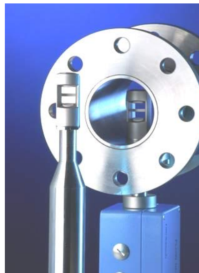
UVA se sondou VA a měřicí trasou VA Di
