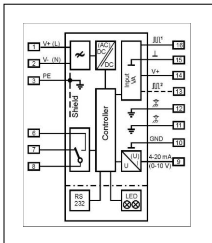
Blokové schéma zapojení převodníku UFA v provedení
