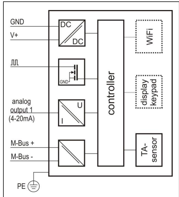
Schema zapojení U10b ve variant s M-bus
