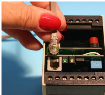
Abb.3 Sicherung TR5
